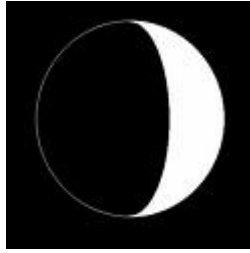
LUNA CRECIENTE
