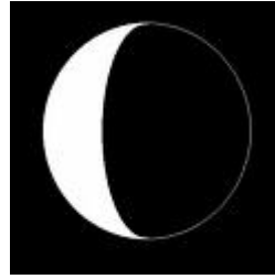
LUNA MENGUANTE
